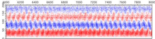
(d) Ra=3 \times 10^4 and Q=8 \times 10^1 : no rolls, fluctuating cell
